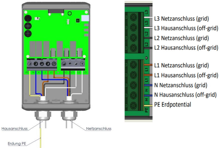
Abb. 7: Netzanschluss mit Kabeldurchführung und Belegung
