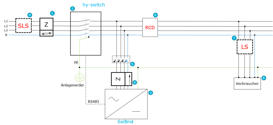
Abb. 6: Einbindung in TT-Netz
