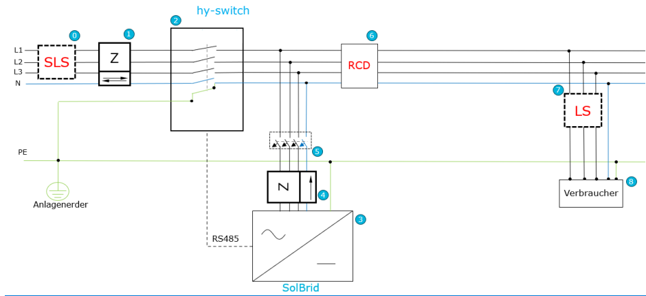
Abb. 5: Einbindung in TN-S-Netz
