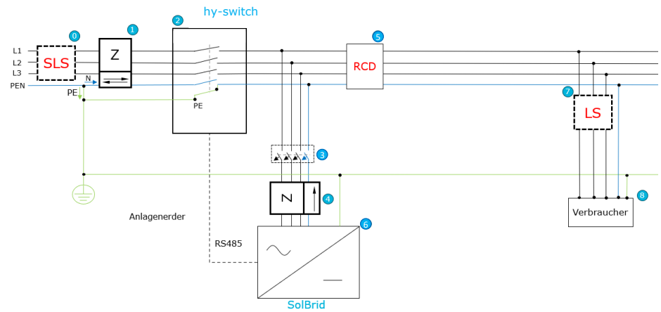
Abb. 4: Einbindung in TN-C-S-Netz
