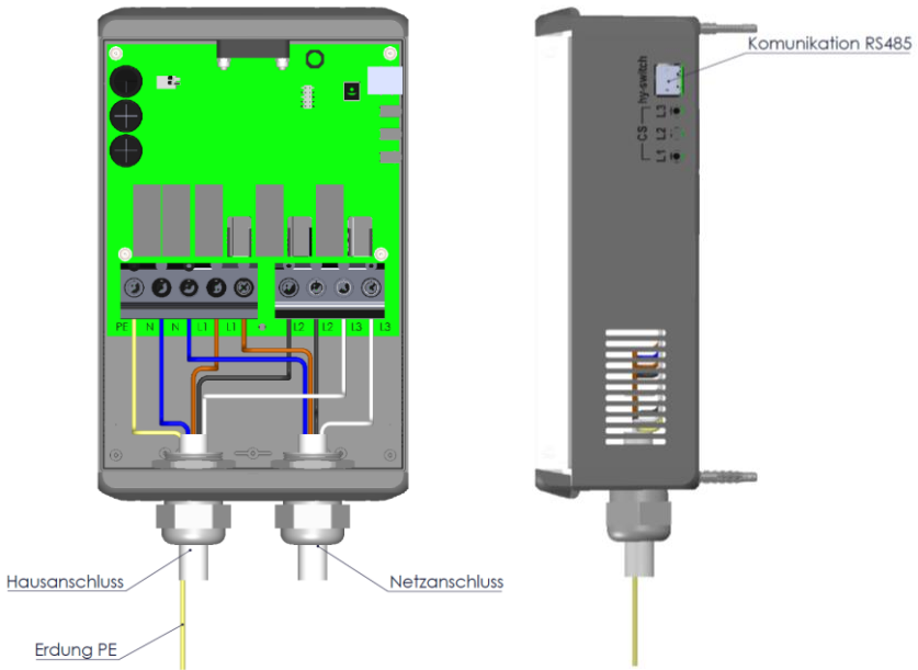
Abb. 2: Aufbau der Komponente mit äußeren Anschlüssen
