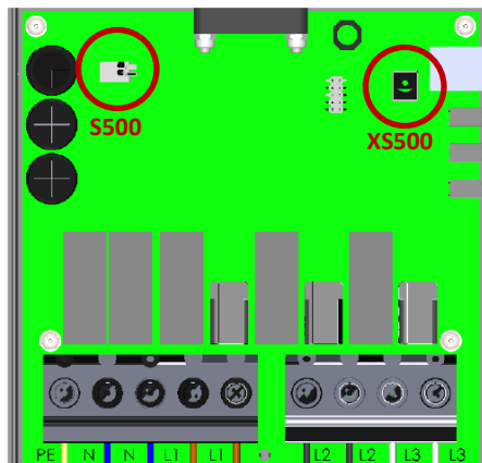
Abb. 9 Rücksetzen der Relais
